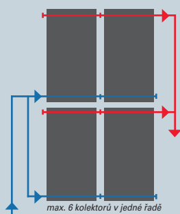
Vertikální (typ FM-S)
